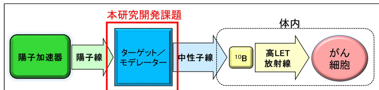
図：加速器型BNCTの模式図
