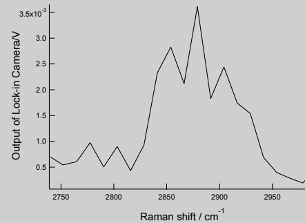
試作したCMOS-SRSイメージャで取得した ステアリン酸の誘導ラマンスペクトル
