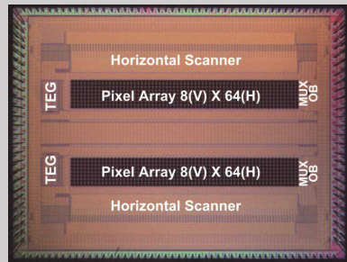
試作したCMOS-SRSイメージャのチップ写真
