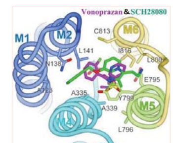
胃プロトンポンプと医薬品複合体構造 (革新的中分子創薬技術の開発)
