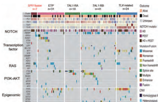
図 3 KMT2Ar-ALL への統合的クラスター
