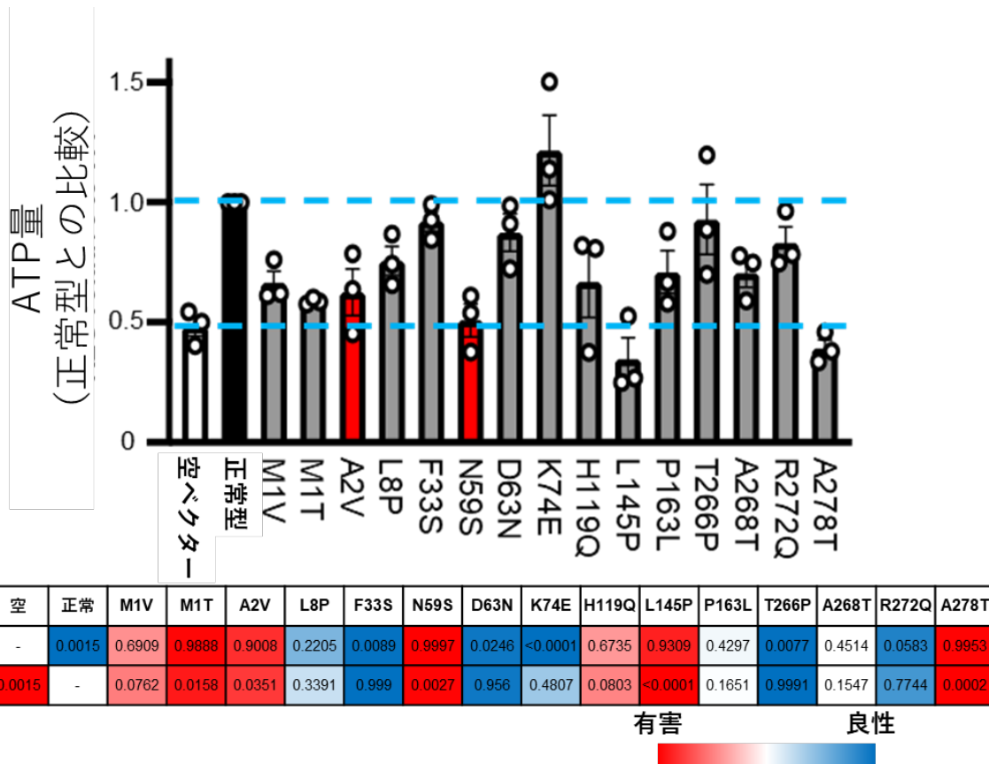
図2. ATP量を指標としたバリエントの簡便かつ網羅的解析
