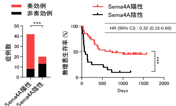
図3. セマフォリン4Aを発現している非小細胞肺がん症例では抗PD-1抗体の治療効果が高い(自験例の解析)
