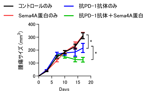
図4. セマフォリン4A蛋白投与は抗PD-1抗体の治療効果を増強する
