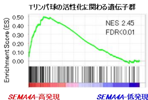
図2. セマフォリン4Aを高発現している非小細胞肺がん症例ではTリンパ球の活性化に関わる遺伝子群の発現が上昇している(がんデータベースの解析)
