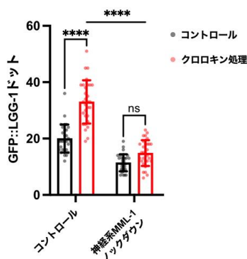
図4. 神経系 MML-1 は遠位組織のオートファジーを制御する
