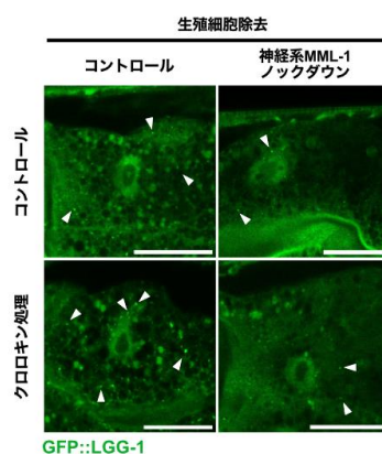
図4. 神経系 MML-1 は遠位組織のオートファジーを制御する
