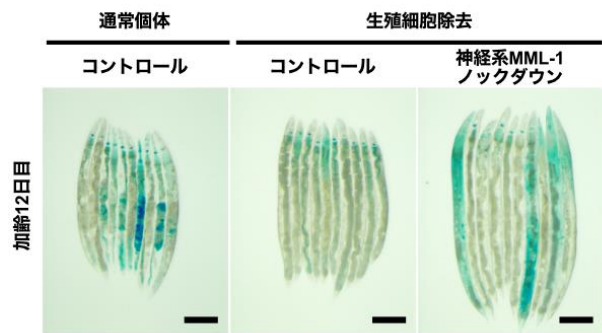
図2. 神経系 MML-1 の抑制により線虫の長寿が廃止される
