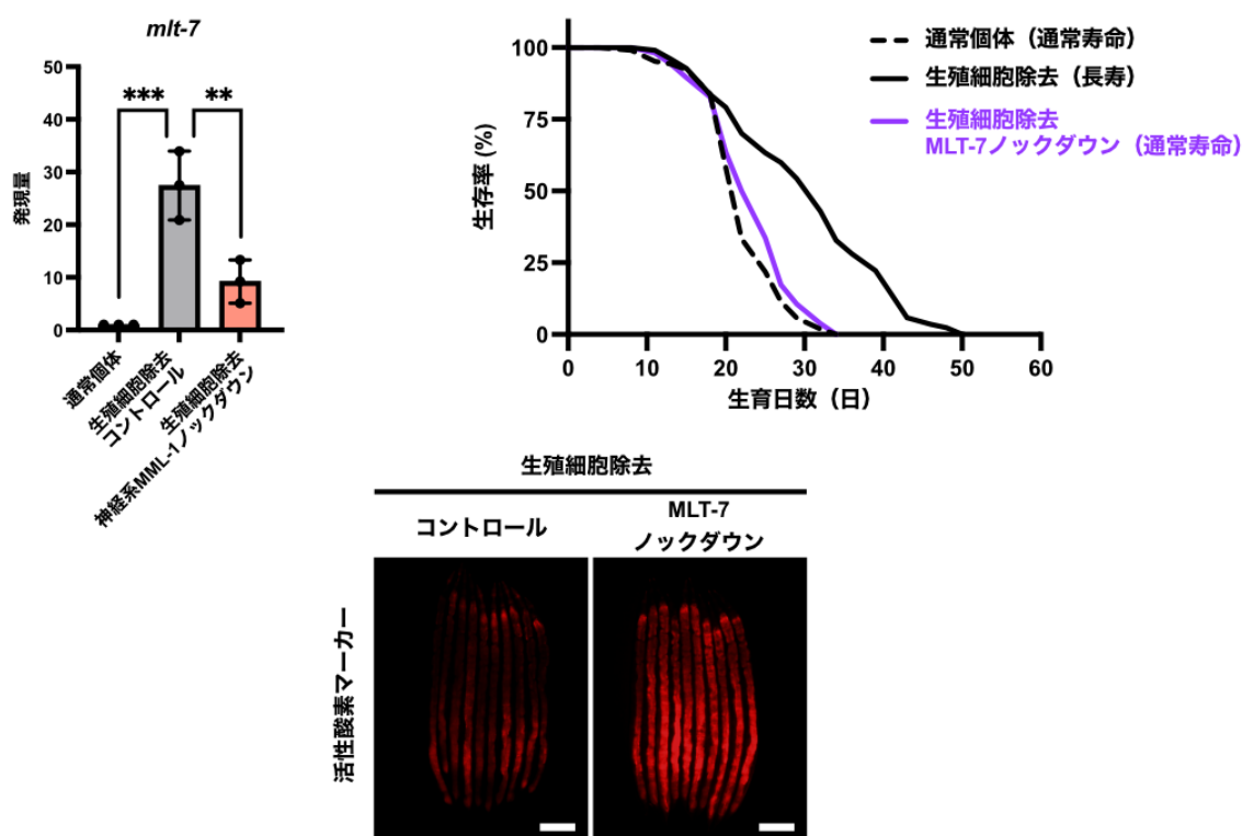
図5. 神経系 MML-1 は MLT-7 を活性化し、活性酸素の蓄積を抑制する
