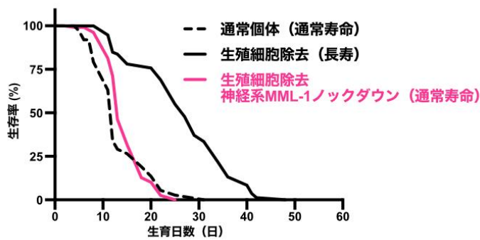
図2. 神経系 MML-1 の抑制により線虫の長寿が廃止される
