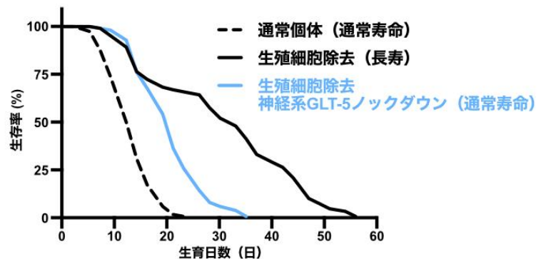
図3. 神経系 MML-1 は GLT-5 を発現上昇させることで寿命を延ばす
