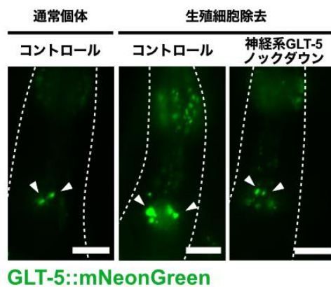
図3. 神経系 MML-1 は GLT-5 を発現上昇させることで寿命を延ばす
