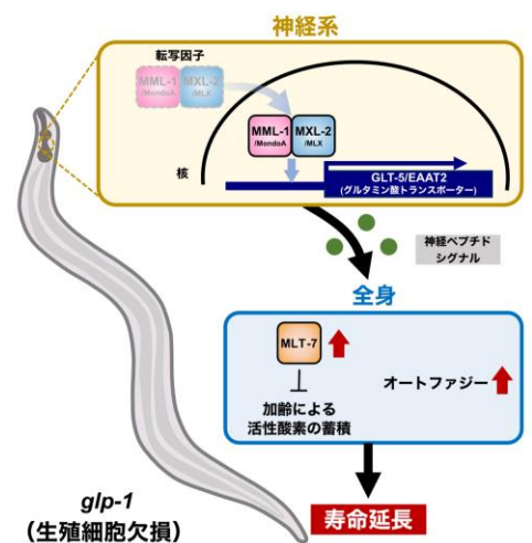
図1. 研究成果概略
