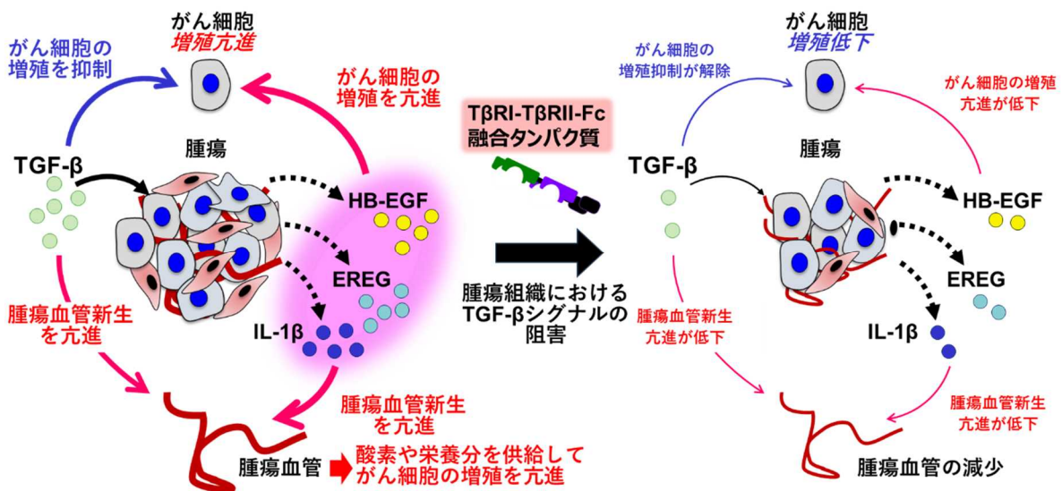
図4 TGF-β 阻害 Fc 融合タンパク質はがん微小環境ネットワークを遮断することで腫瘍形成を阻害する がん微小環境における TGF-β シグナルは、がん細胞の増殖を抑制するが、同時にがん細胞やがん間質などに作用して HB-EGF などの、がん細胞の増殖や腫瘍血管新生を亢進する因子の発現を上昇させることで間接的にがん細胞の増殖を亢進する (図左)。TGF-β 阻害 Fc 融合タンパク質 (TβRI-TβRII-Fc) は、腫瘍組織における TGF-β シグナルを阻害して HB-EGF などの発現を低下させることで、がん微小環境ネットワークが遮断され、がん細胞の増殖の低下や腫瘍血管の減少を介して、結果として腫瘍形成が阻害されることが明らかとなった。
