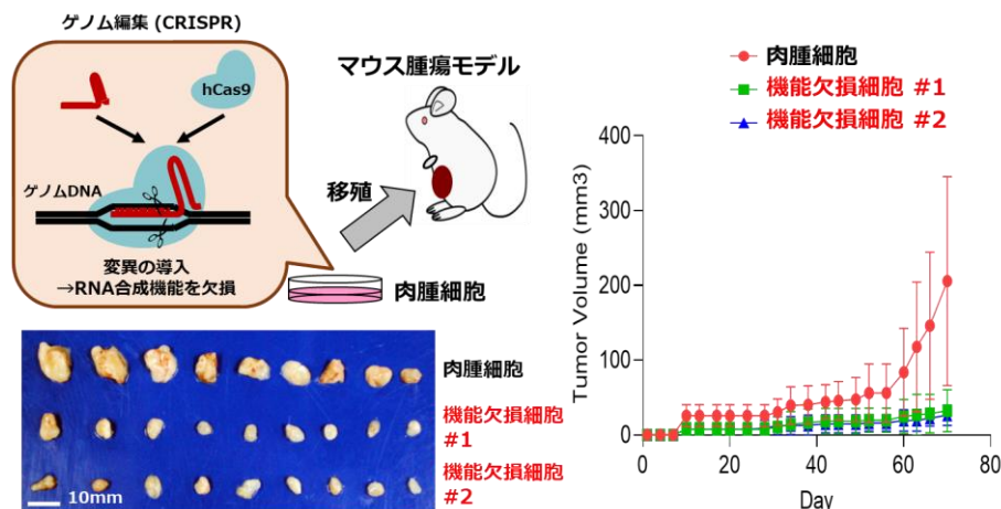
図 4 テロメラーゼ逆転写酵素(hTERT)の新たな機能をおさえた肉腫細胞の解析
