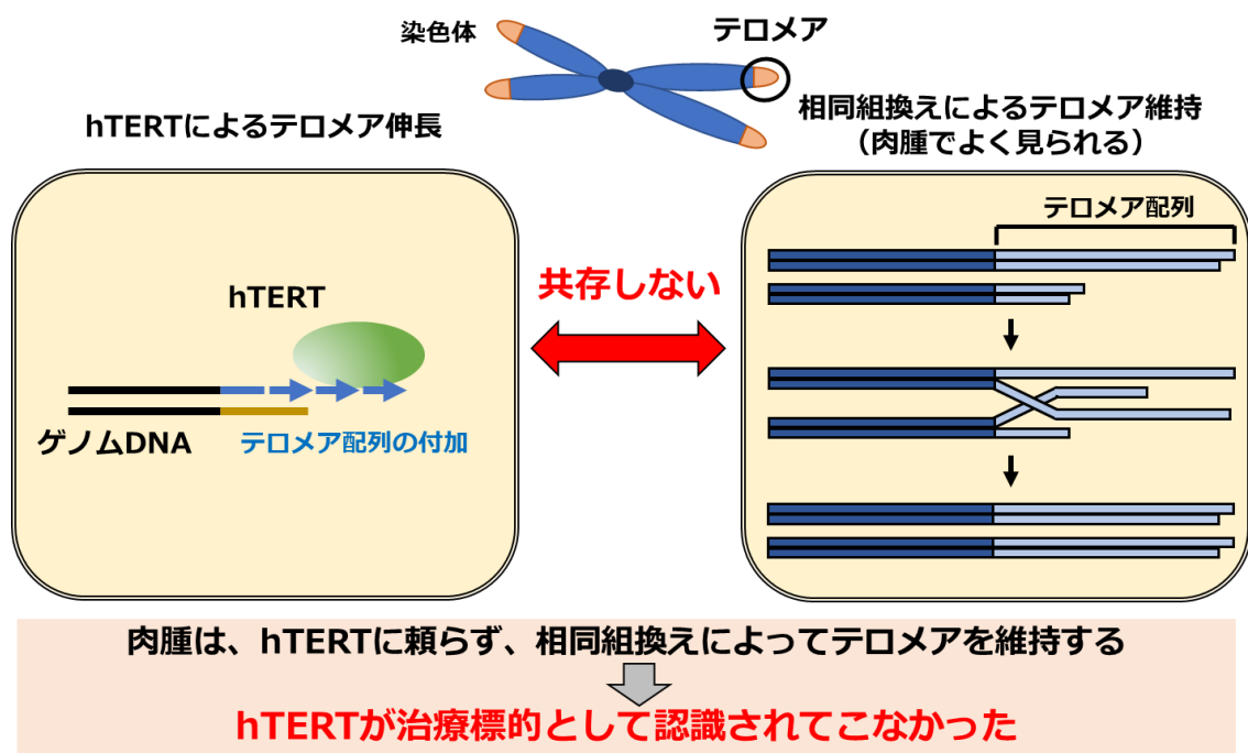
図 2 テロメアを維持する仕組み
