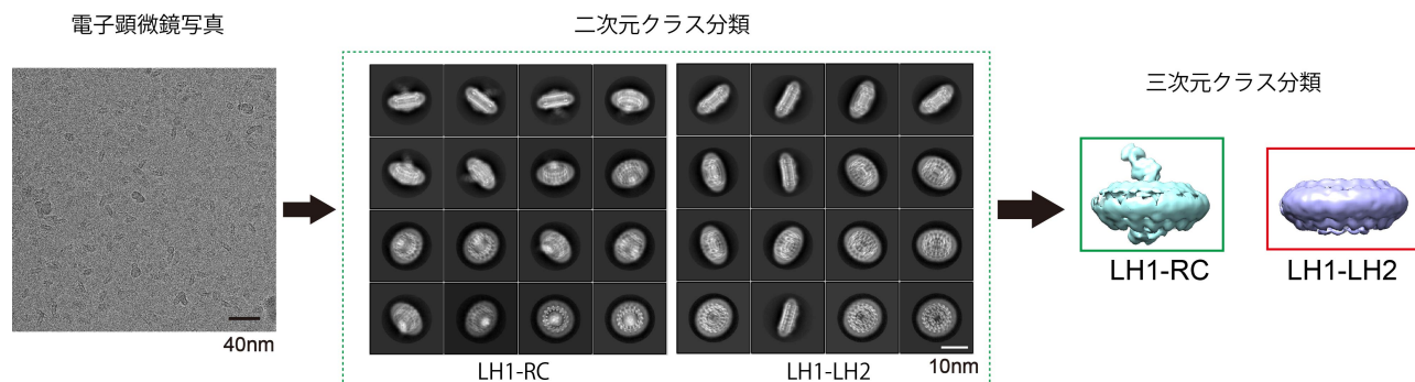
図1 クライオ電子顕微鏡写真から計算機により分類可視化された Hlr. halophila のコア光捕集反応中心複合体 (LH1-RC) と光捕集共複合体 (LH1-LH2)。クライオ電子顕微鏡写真 (左図) から二次元クラス分類 注10) 後の平均化された投影像 (中図) は、LH1-RC と LH1-LH2 に分けて表示している。立体構造を基にした三次元クラス分類 注9) により2つの立体構造 (右図) に収束した。
