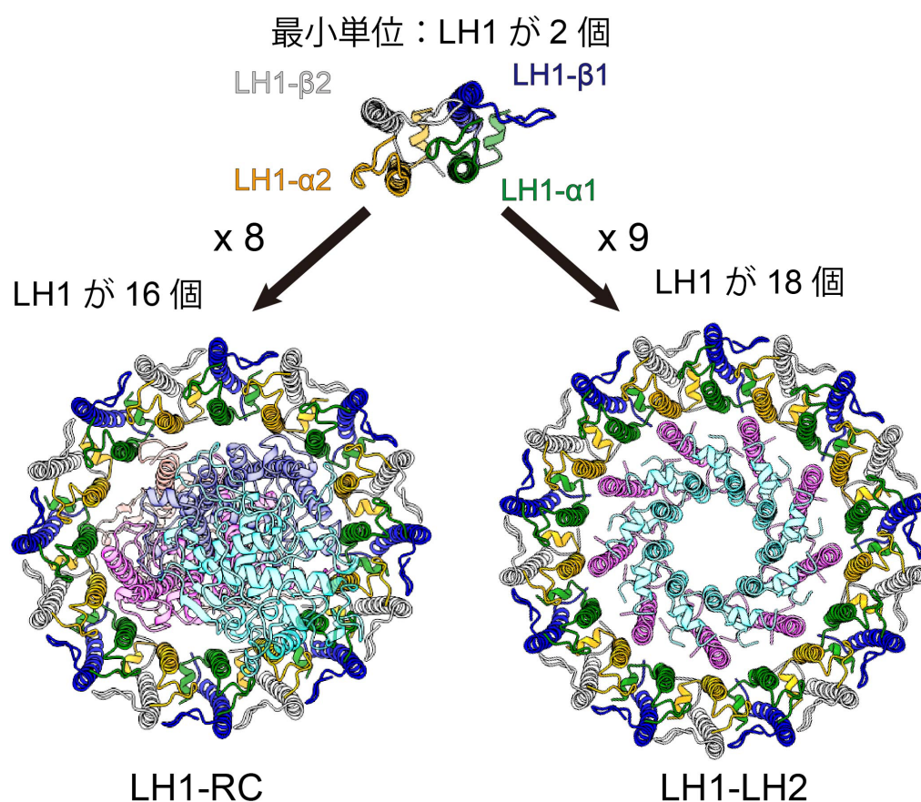
図2 クライオ電子顕微鏡により可視化された Hlr. halophila のコア光捕集反応中心複合体 (LH1-RC) と光捕集共複合体 (LH1-LH2) の立体構造。LH1 サブユニットの \alpha 、 \beta 鎖のそれぞれ2種類のアイソフォーム 注10) がペアとなって、リングの最小構造単位を形成している様子を図示化した。LH1 リングが RC と LH2 (半透明色部分) をそれぞれ取り囲むように並んでいる。
