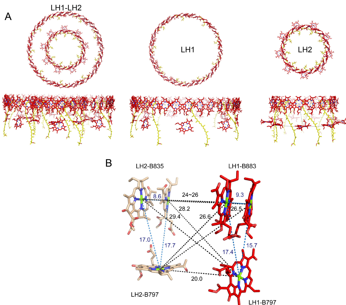
図3 LH1-LH2 共複合体中の色素分子配置
