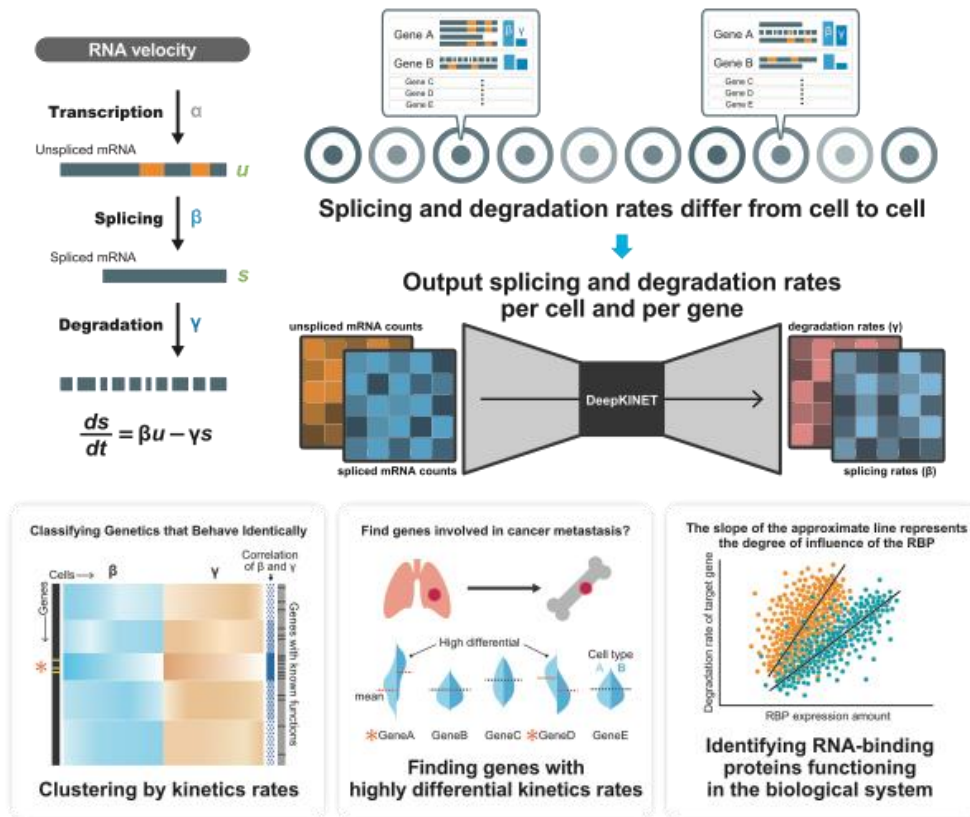
図1 DeepKINET の概要
