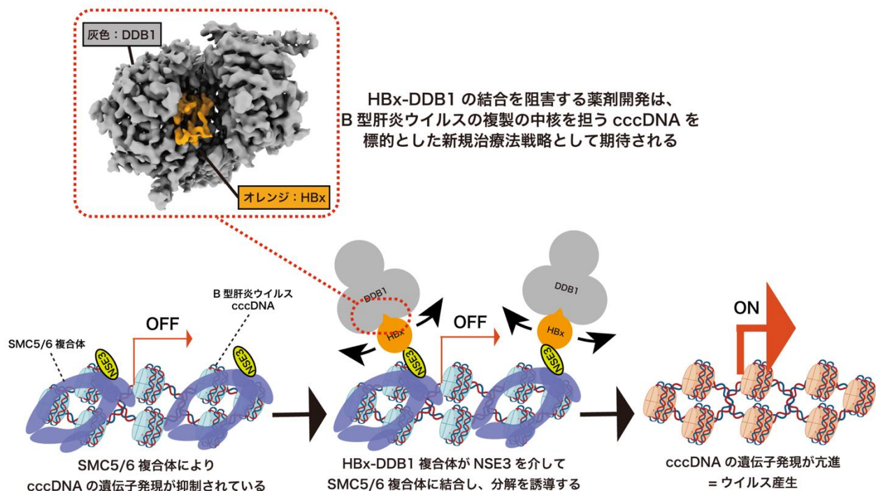
図3 HBx-DDB1複合体によるB型肝炎ウイルス遺伝子発現亢進のモデル
