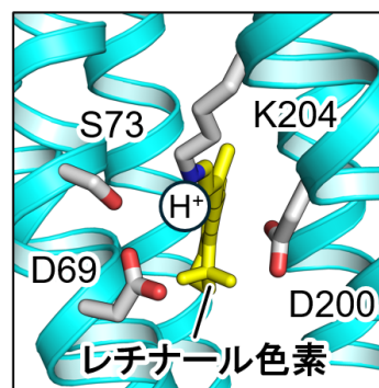
可視光吸収型のレチナール色素に結合している水素イオン ( H^+ ) が紫外吸収型のアプソモナドロブシンでは解離することによって、レチナールの吸収が紫外光の領域にシフトすると考えられる
