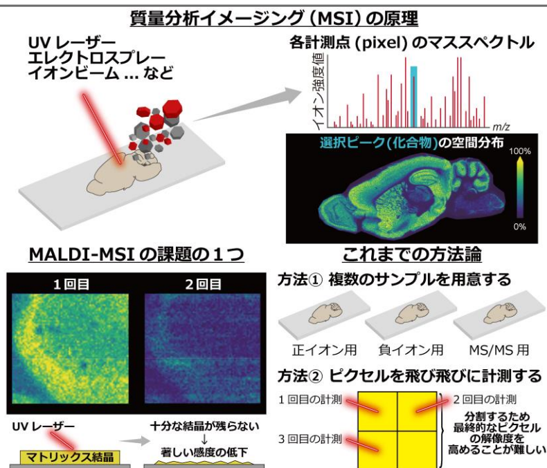
図 2 質量分析イメージングの原理と MALDI-MSI の課題
