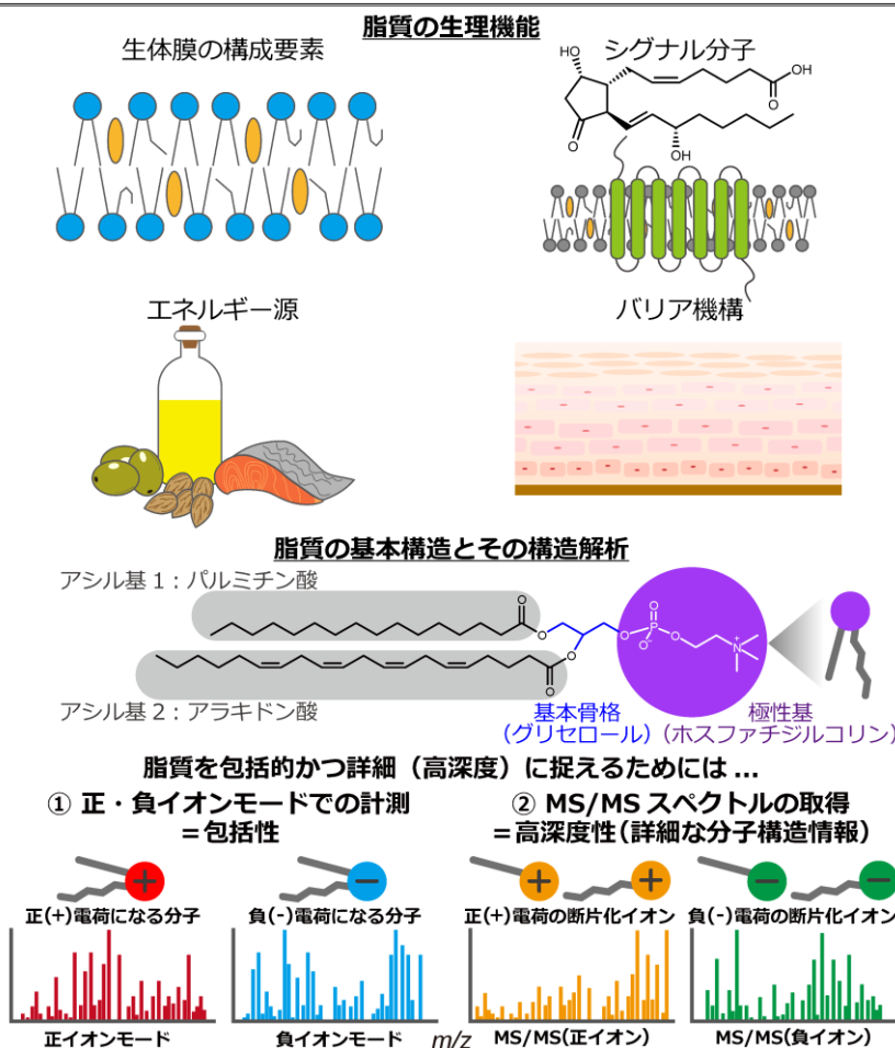
図 1 脂質の生理機能と質量分析を用いた脂質の構造解析 (リポミクス)
