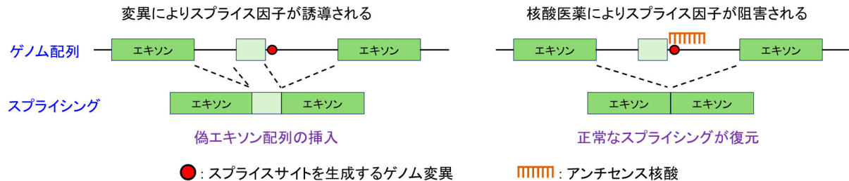
図 2: スプライスサイト生成変異の例。イントロン領域中の変異によりスプライス因子が新規に形成され、新しいエキソン（偽エキソン）が転写配列に挿入されます（左図）。この変異に対する核酸医薬を投与することで、スプライス因子が阻害され、正常なスプライシングが回復します（右図）。
