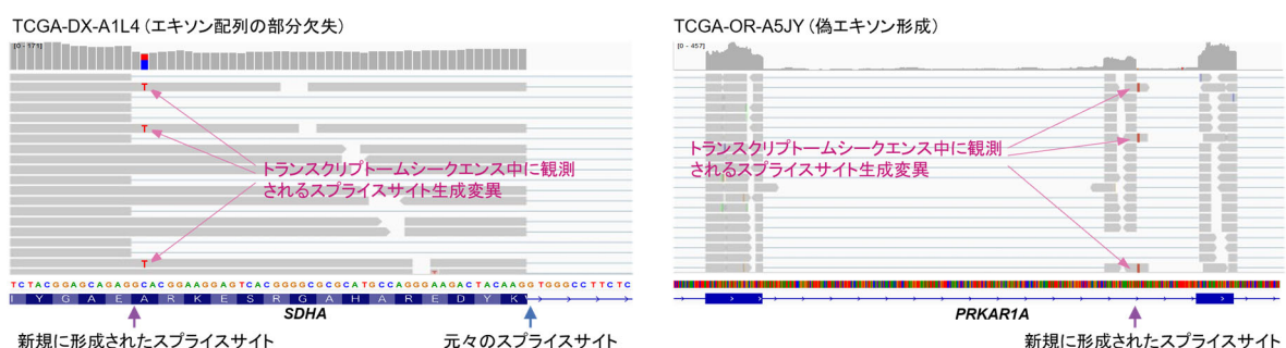
図 3: スプライスサイト生成変異周辺のトランスクリプトームシーケンスのアラインメント図。データ中からスプライスサイト生成変異を観測できるという現象に着目することで、juncmut のアルゴリズム開発へと繋がりました。
